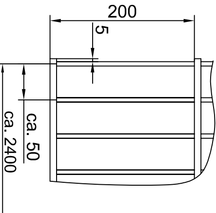
Einzelheit Z
